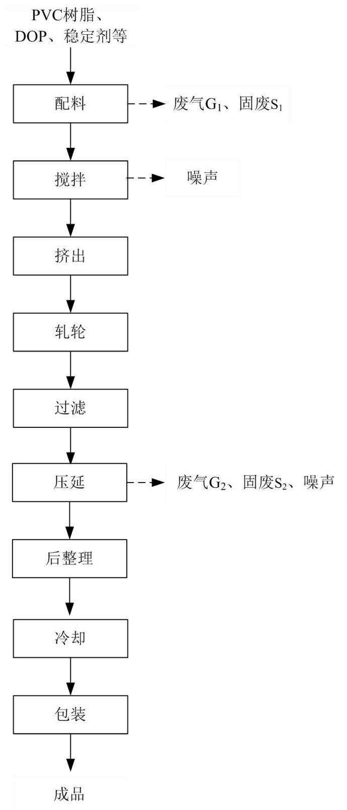
图1-1 PVC压延膜工艺及产污环节
