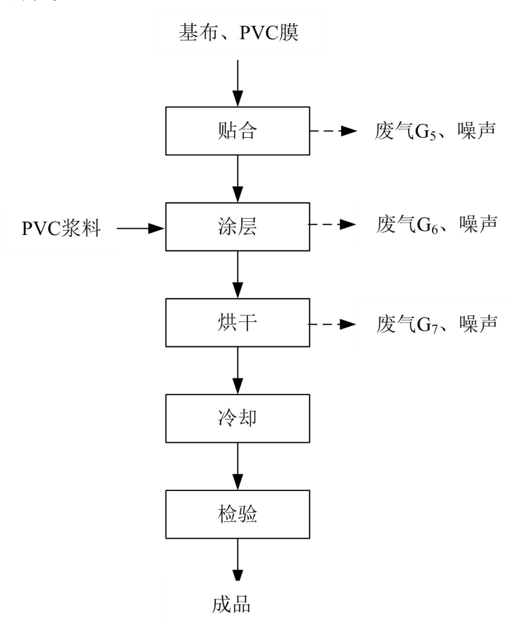
图1-3-2 篷盖材料工艺及产污环节
