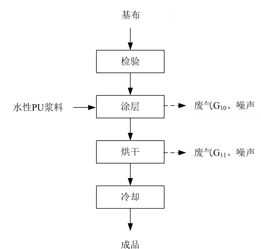
图1-4-2 高档灯箱布工艺及产污环节
