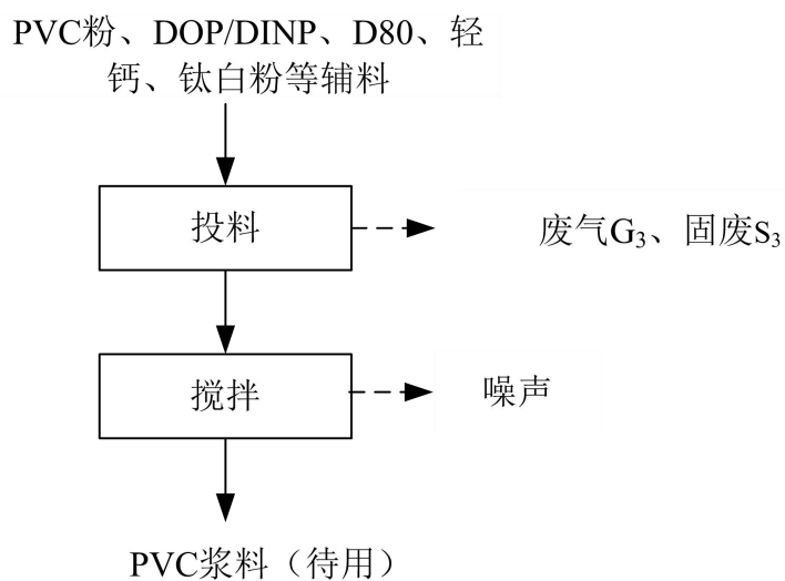
图1-3-1 PVC浆料制备工艺流程及产污环节
