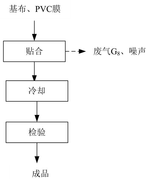
图1-3-3 篷盖材料工艺及产污环节
